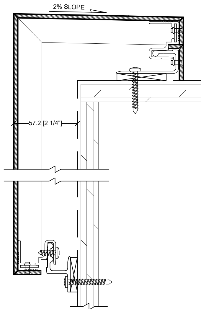
CAP DETAIL TYP.
